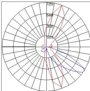
DS323FC-3M-30-T2-600M
